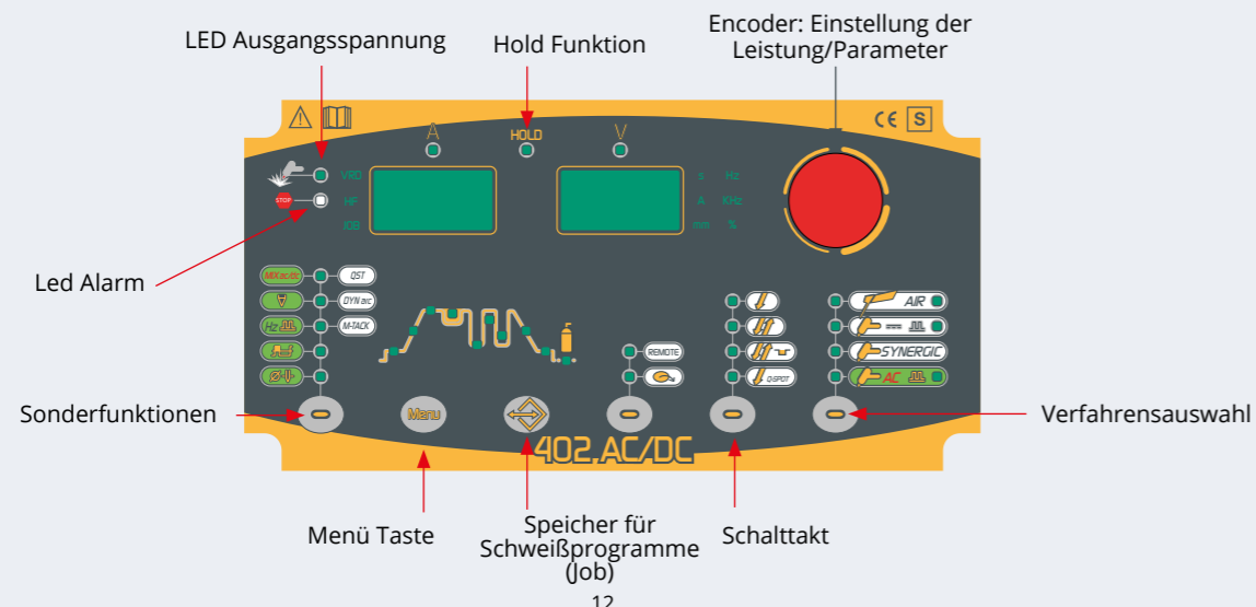
Frontbedienfeld Generator
