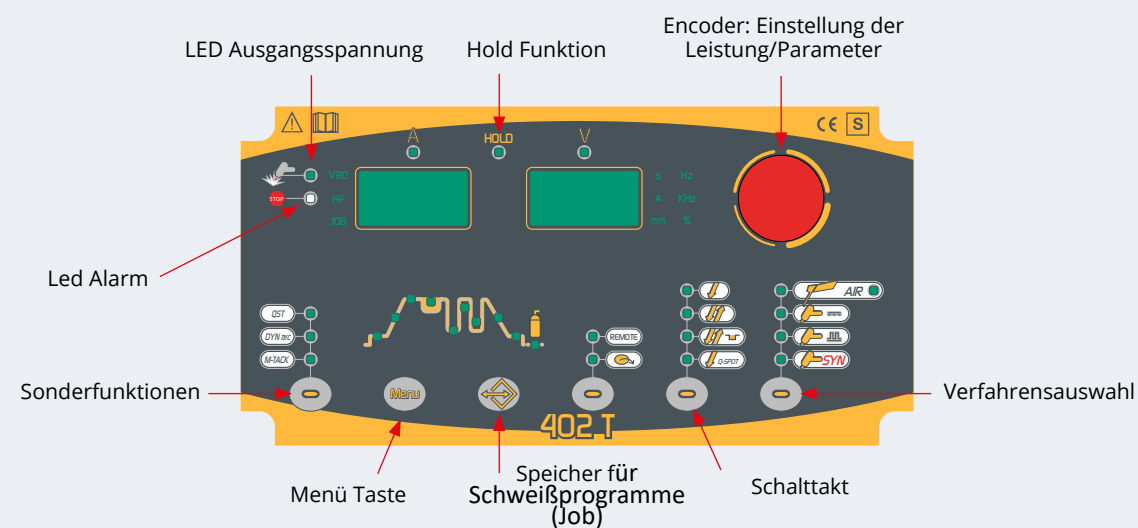
Frontbedienfeld Generator
