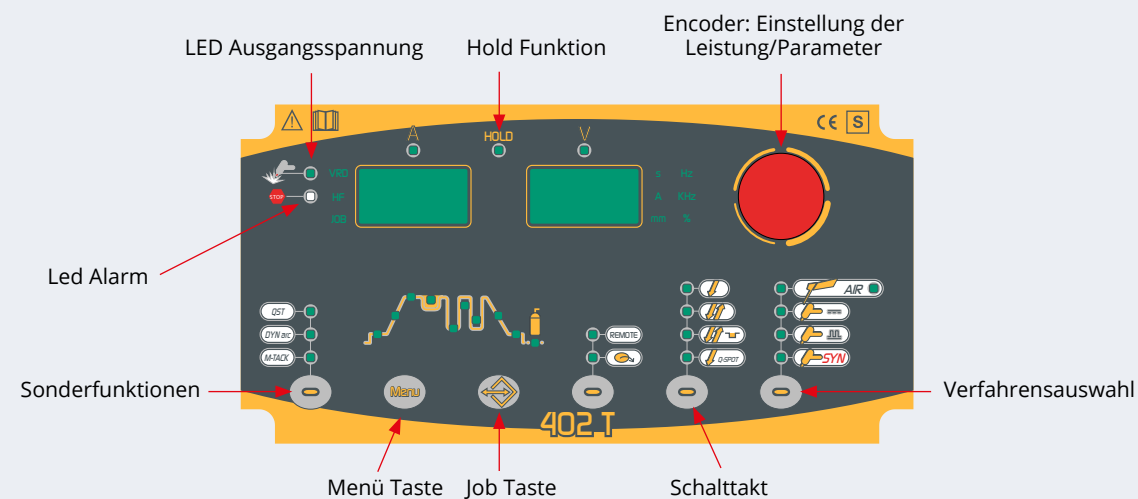
Frontbedienfeld Generator
